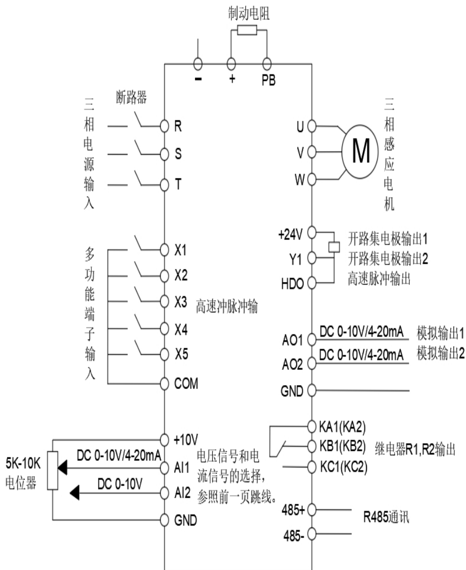
图2-2变频器控制回路接线方式
