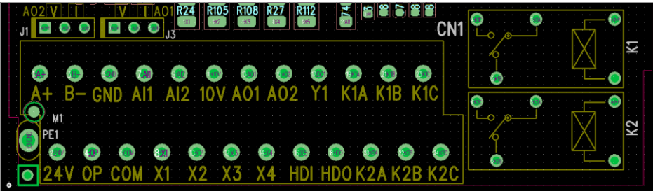
图 2-4 变频器（隔离版本）控制回路端子布置图
