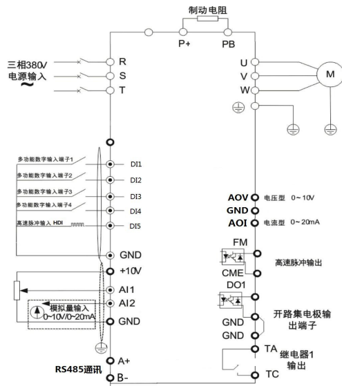
图 2-2 变频器控制回路接线方式
