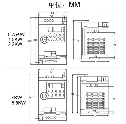
图 1-1 塑胶结构外型尺寸及安装尺寸示意图
